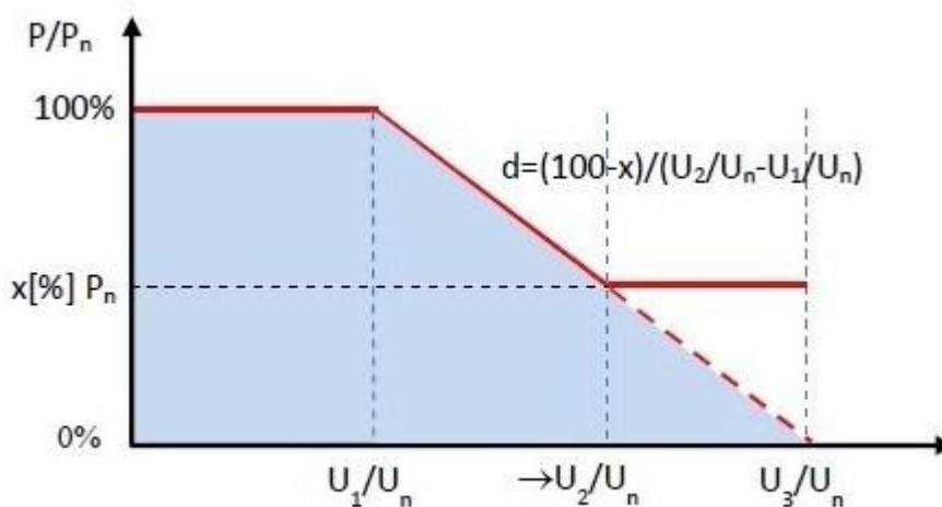
Obrázek 8: Charakteristika funkce P(U)
