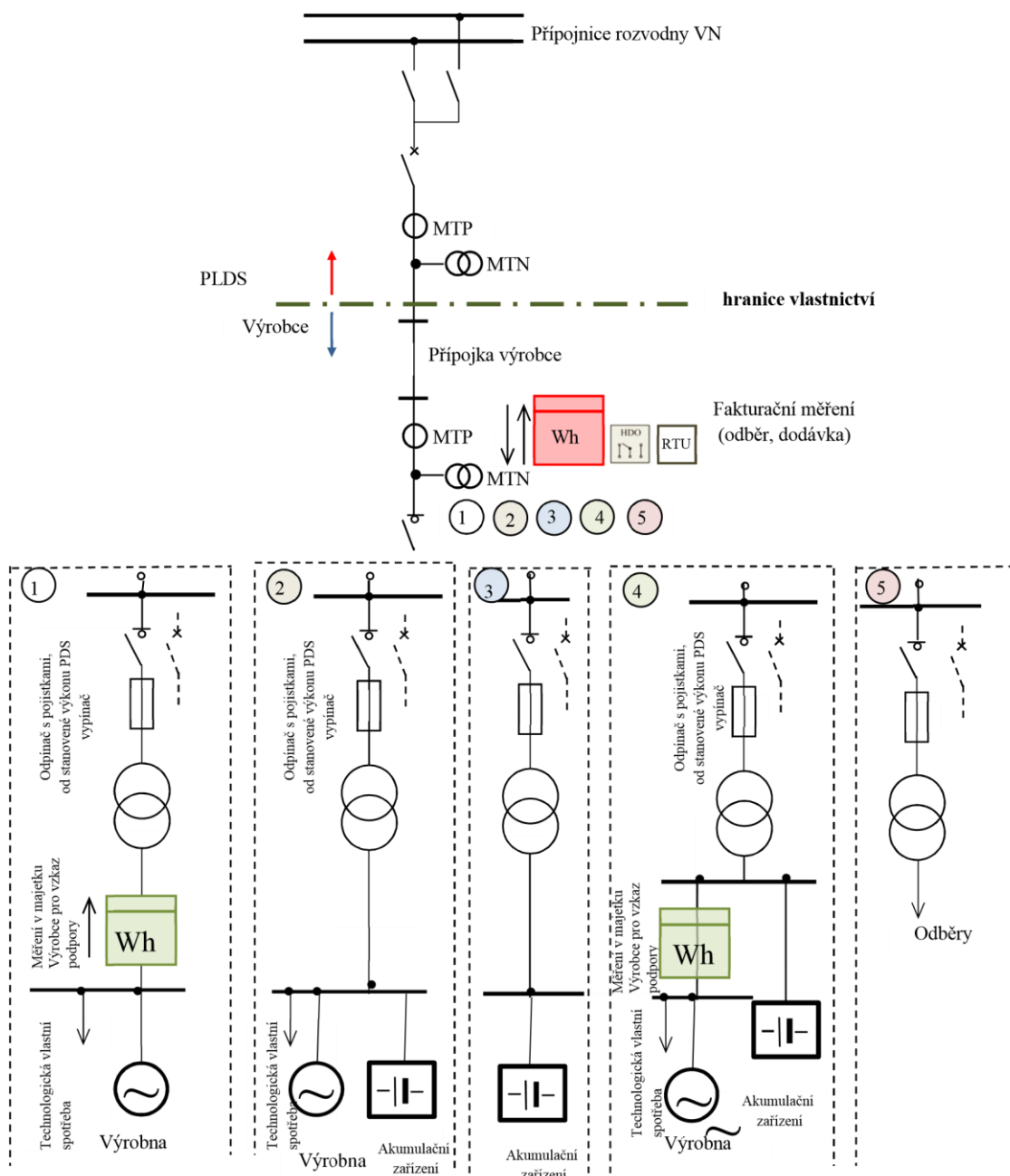
Obrázek 13: Připojení výroby elektřiny a akumulčního zařízení samostatným vedením do vn rozvodny LDS
