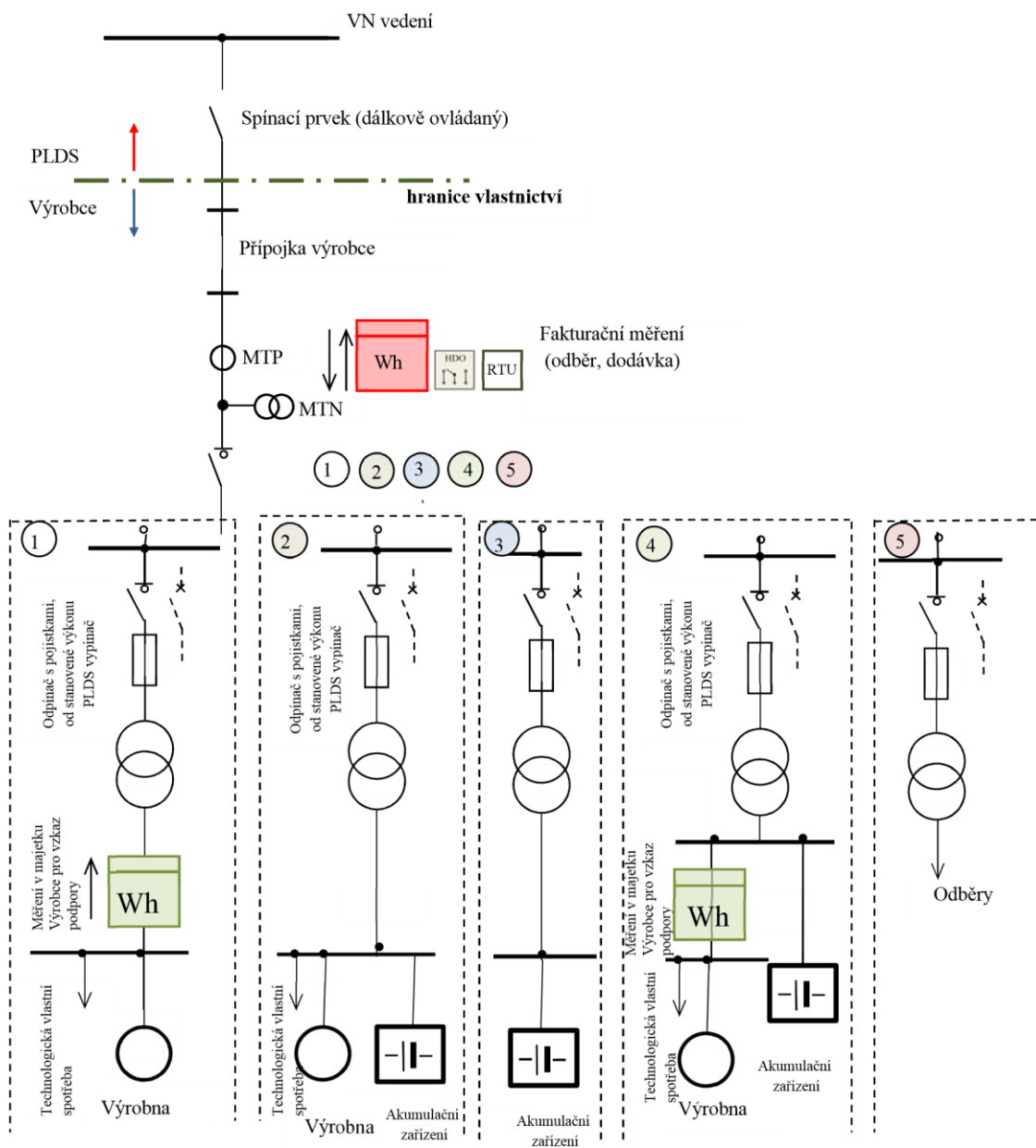
Obrázek 12: Připojení výroby elektřiny a akumulčního zařízení z nadzemního vedení vn přípojkou výrobce
