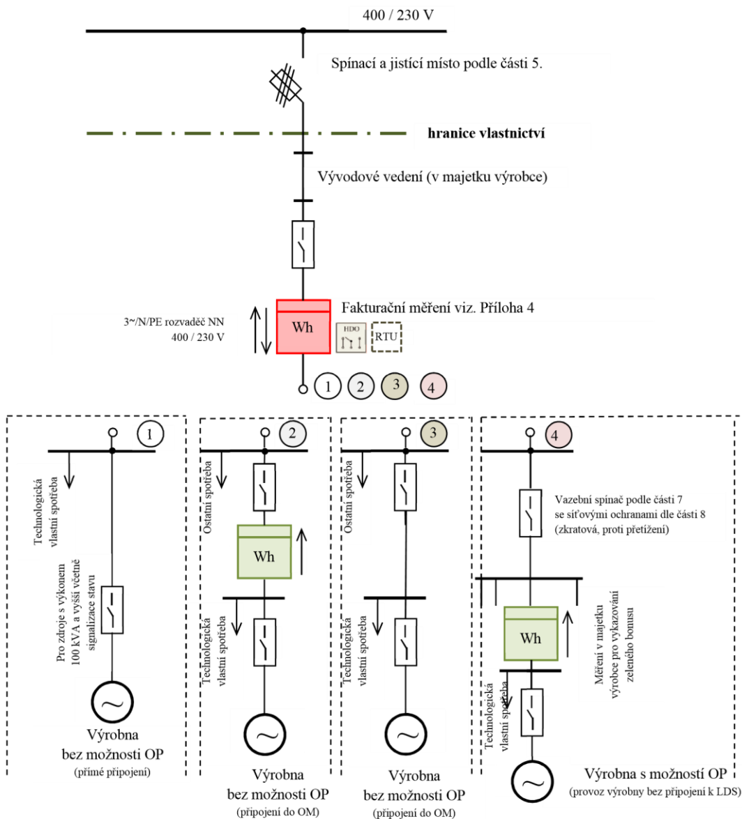
Obrázek 10: Připojení výroby elektřiny do nn
