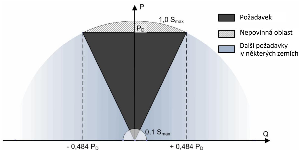
Obrázek 1: Požadavky na dodávku/odběr jalového výkonu při jmenovitém napětí
