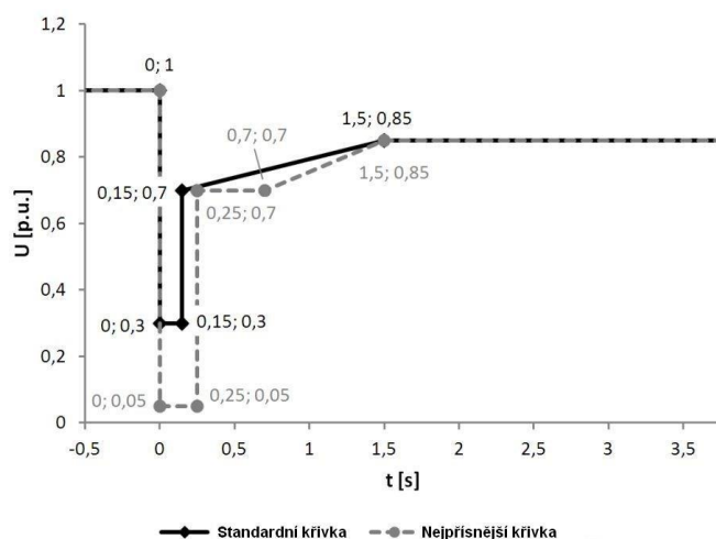
Obrázek 3: Schopnost překlenutí poruchy přímo připojených generátorů
