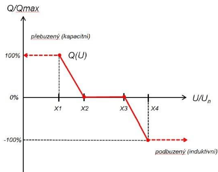
Obrázek 9: Charakteristiky funkce Q(U)
