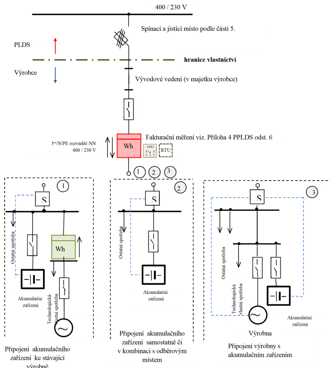
Obrázek 11: Připojení výrobní elektřiny s akumulčním zařízením do nn
